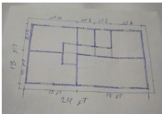
Grondtekening van het huis.
